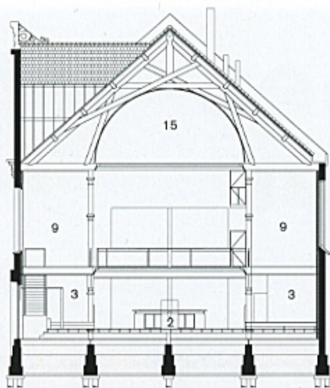
Dwarsdoorsnede
