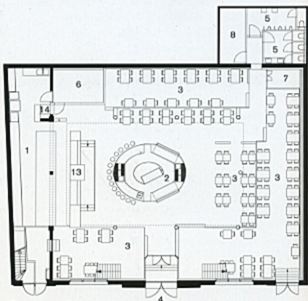
Begane grond
