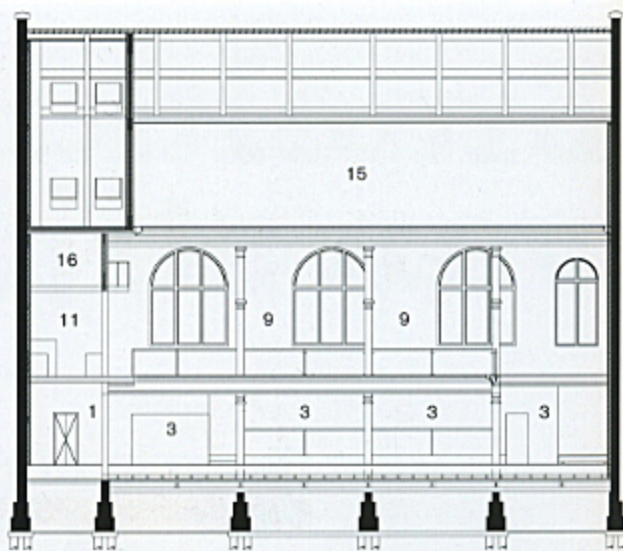
Langsdoorsnede
